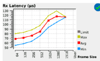
Die Verzögerung (Latency) liegt unter 120 µsec
