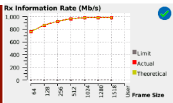
Die Messung der Datenübertragung zeigt eine optimale Performance (RFC 2544 Test mit UniPro GIG)
